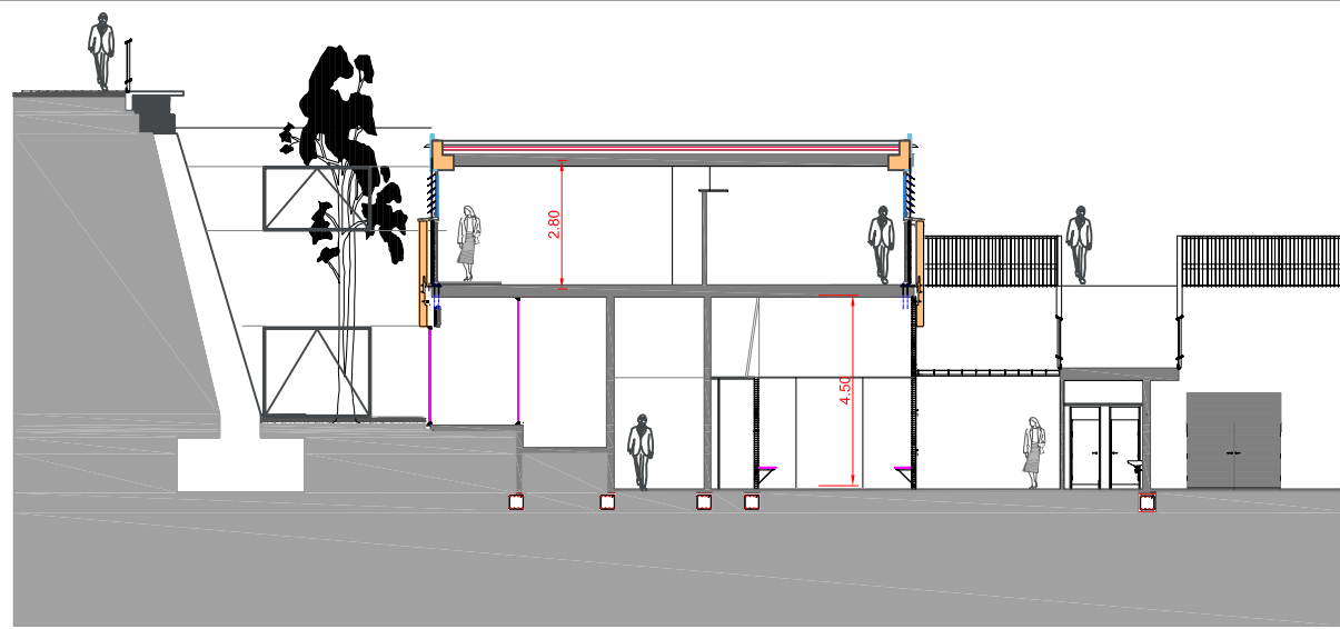
SECCIÓ G-G
