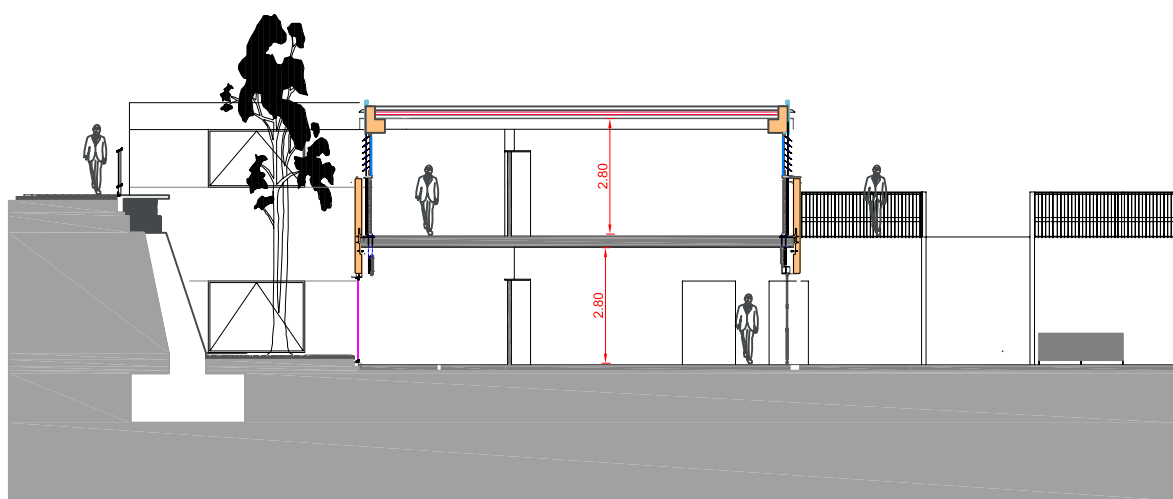
SECCIÓ K-K
