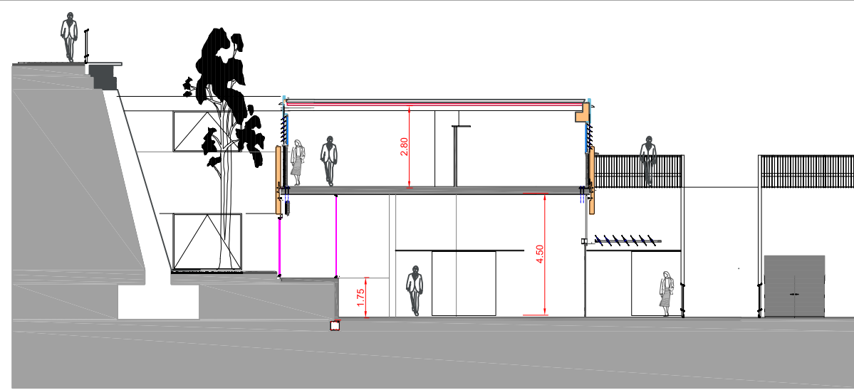
SECCIÓ H-H
