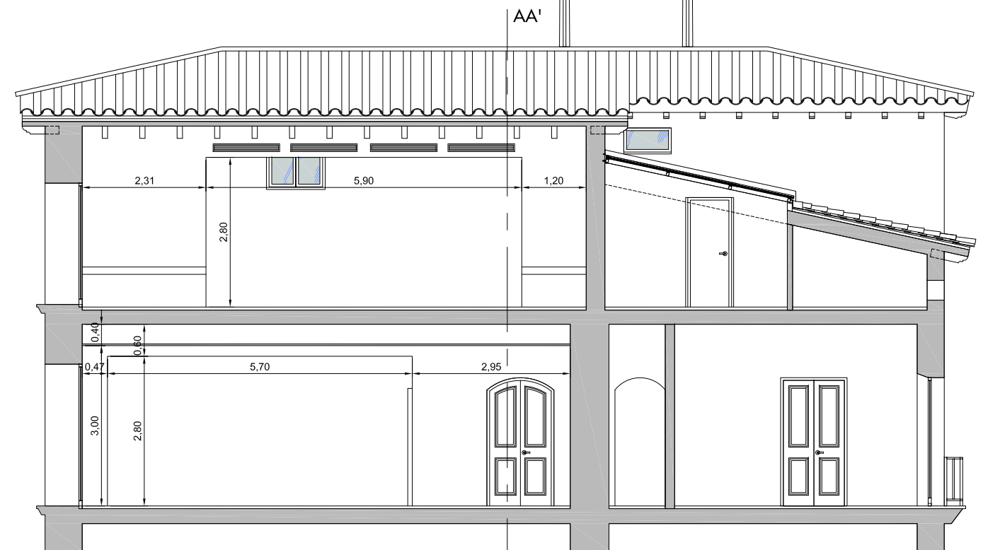
Secció BB' (e: 1/100)
