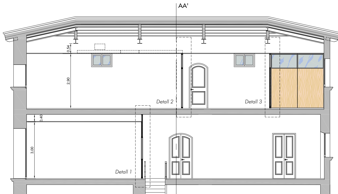
Secció CC' (e: 1/100)
