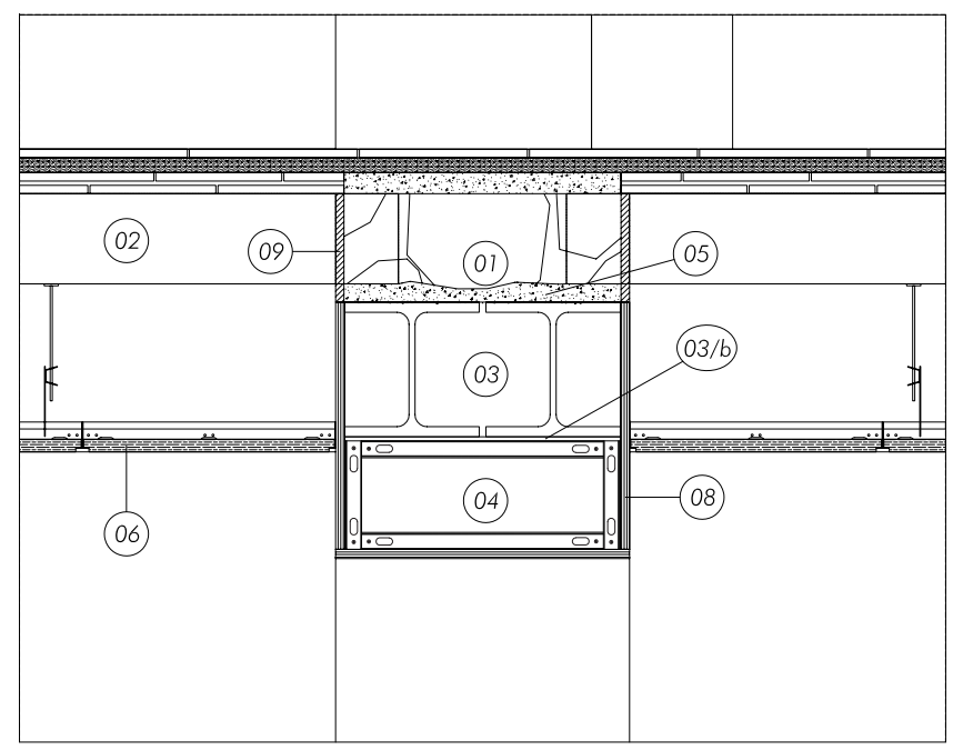
Detall 1 (e: 1/20)
