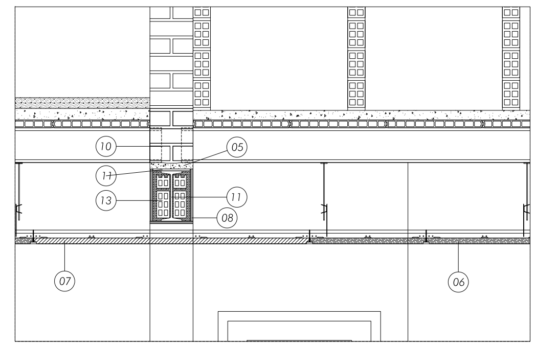
Detall 2 (e: 1/20)
