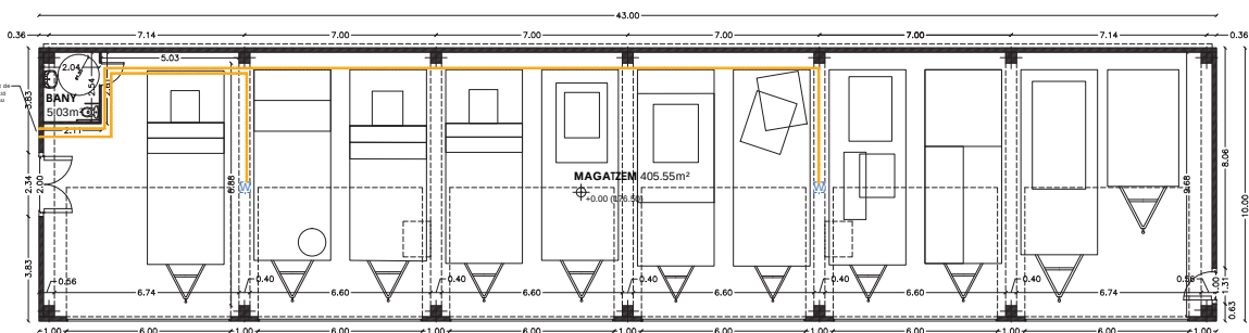
PLANTA BAIXA
