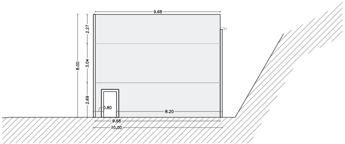
ALÇAT FAÇANA LATERAL 2
