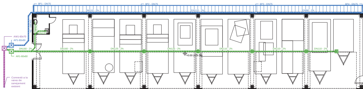
PLANTA BAIXA
