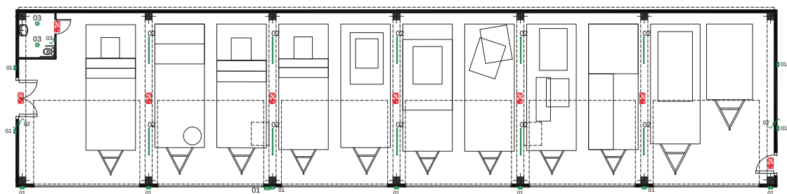
PLANTA BAIXA
