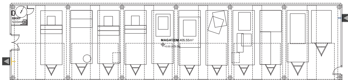
PLANTA BAIXA
