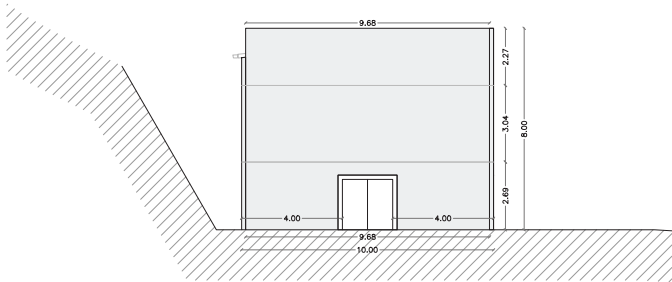
ALÇAT FAÇANA LATERAL 1
