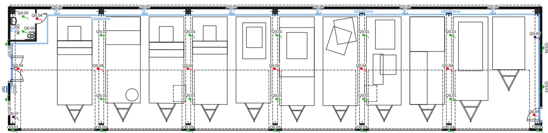
PLANTA BAIXA
