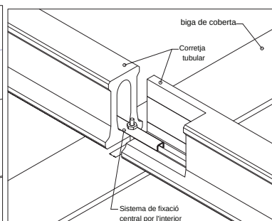
SISTEMA FIXACIÓ STANDARD CORREAS CENTRALS
