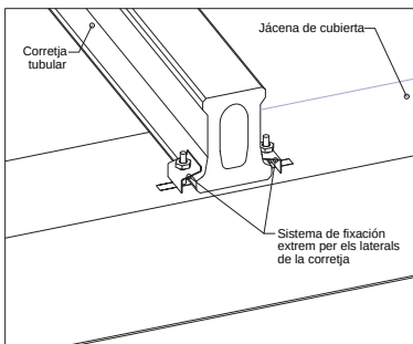
SISTEMA FIJACIÓN STANDARD CORREAS EXTREMAS
