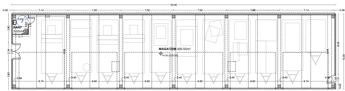
PLANTA BAIXA
