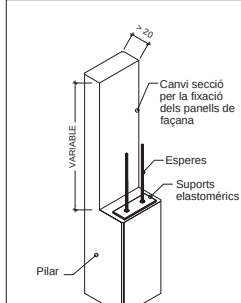
CAP DE PILAR AMB CANVI SECCIÓ AMB ESPERES
