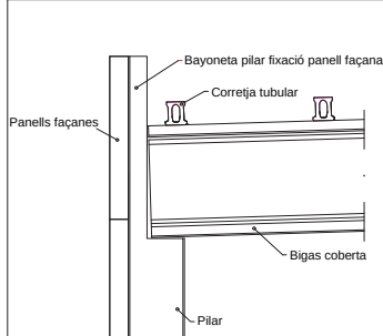
DETALL TROBADA PILAR I BIGA
